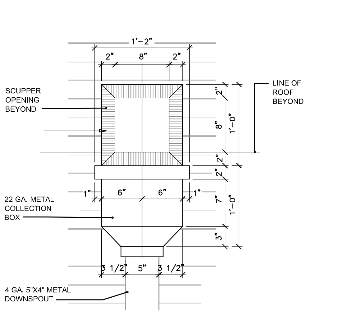
7 A502 NTS DET1
